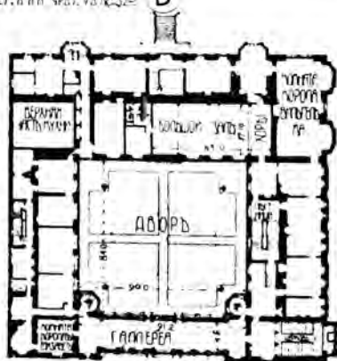
Д ЗАМОКЪ АШБИ (CASTLE ASHBY) ПЛАНЪ II ЭТАЖА
