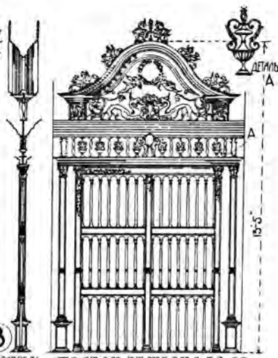
ЖЕЛЪЗН-РЪШЕТКА ВЪ СОВО- РЬ ВЪ СІГУЭНСЬ.
