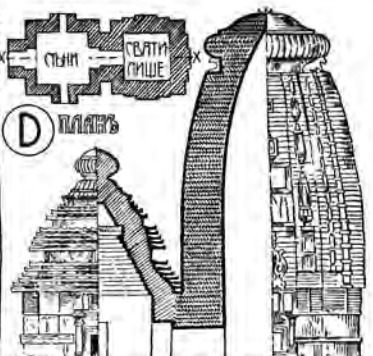
Д ПЛАНЪ Е Желсда и Жазрвзя по X-XI вѣкамъ въ Калаярукъ въ обл. Орхеса. Типичн. образецъ храма - квадратно въ планѣ святилище имѣеть видъ суживающейся вверху башни или стѣны, увѣнчанной амаллою
