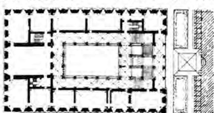
Е ПЛАНЪ II ЭТ.
