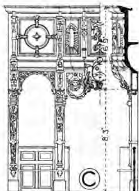
СЪ ФРАСАДА ПЕРЕГРАДА ВЪ ЦЕРКВИ
