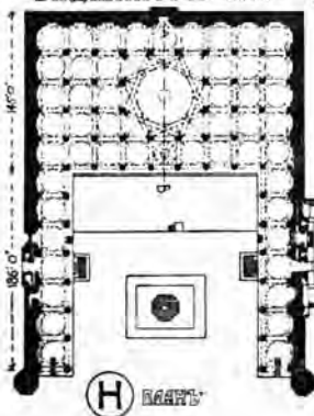
ГЛАВНАЯ МЕЧЕТЬ въ БИДЖАПУРЪ - XVI вѣ.
