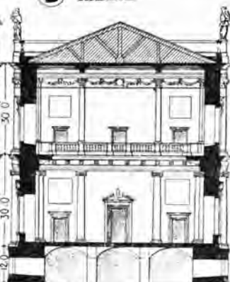
D РАЗРѢЗЪ
