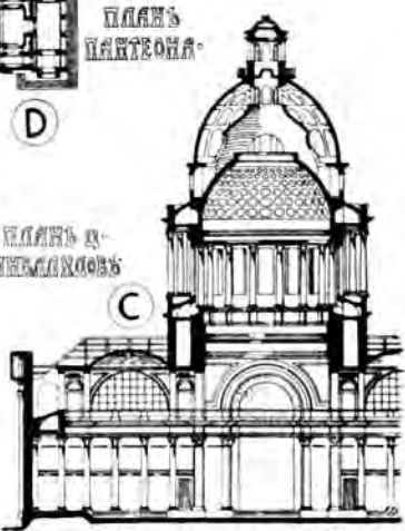
РАЗРЕЗЪ КУПОЛА ПАВТРОНА ВЪ ПАРИЖЕ - 1733-1781 г.; 304Ч. СУФЛО
