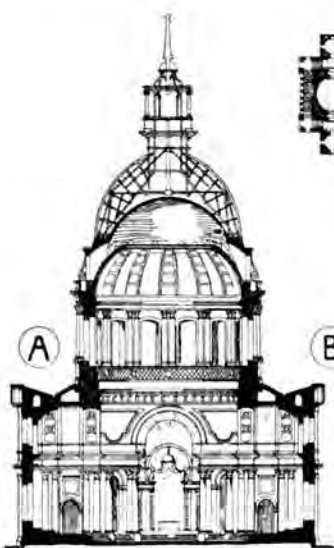
РАЗРЕЗЪ КУПОЛА СЪ КИВЛА - 304Ч. Ж. ДЕВИЛЬЕ ВЪ ПАРИЖЕ - 1670-1706 г.; МАНСАРЪ
