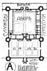
ЗАМОКЪ ШАМБОРЪ • 3047-ШЕРЪ НЕВЪ (NEVEU) • 1526 г.
