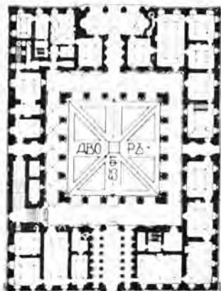
F ПЛАНЪ I-го ЭТАЖА
