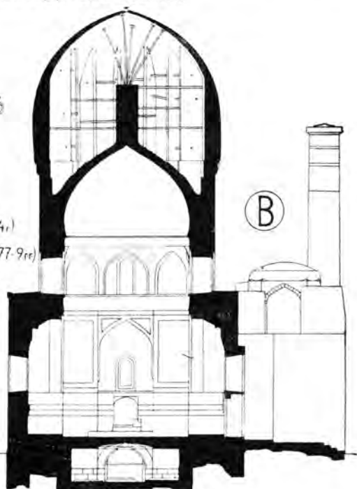
РАЗРѢЗЪ ПО ПЛАНУ А-Б.
