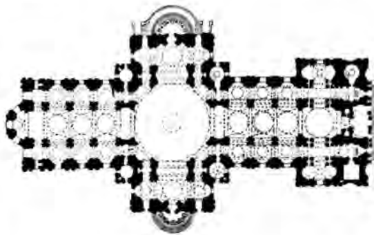
(A) СОБОРЪ СВ. ПЕТРА ВЪ ЛОНДОНѢ 1575 Г. МАШТ. 1:1100
