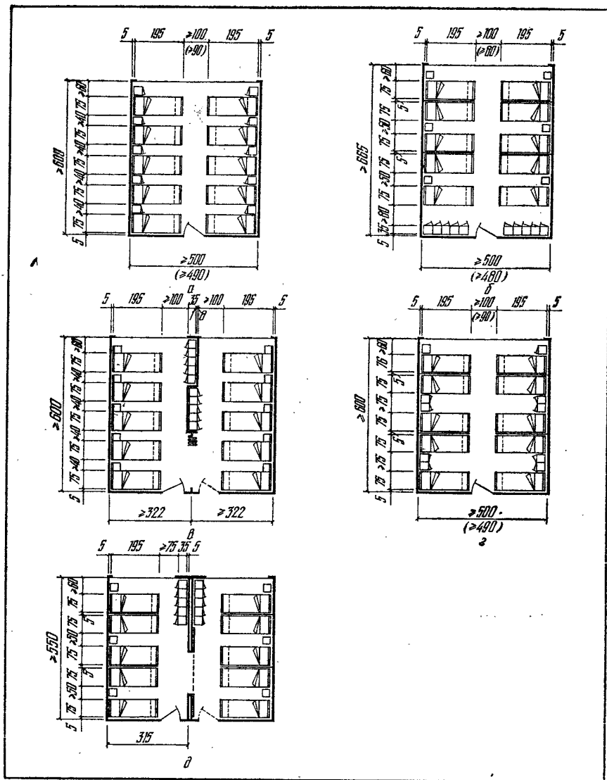
Рис. VII.110. Габариты спальных комнат на 10 мест для пионеров и октябрят в неотпливаемых (в скобках) и отапливаемых павильонах и зданиях с расположением шкафчиков:
