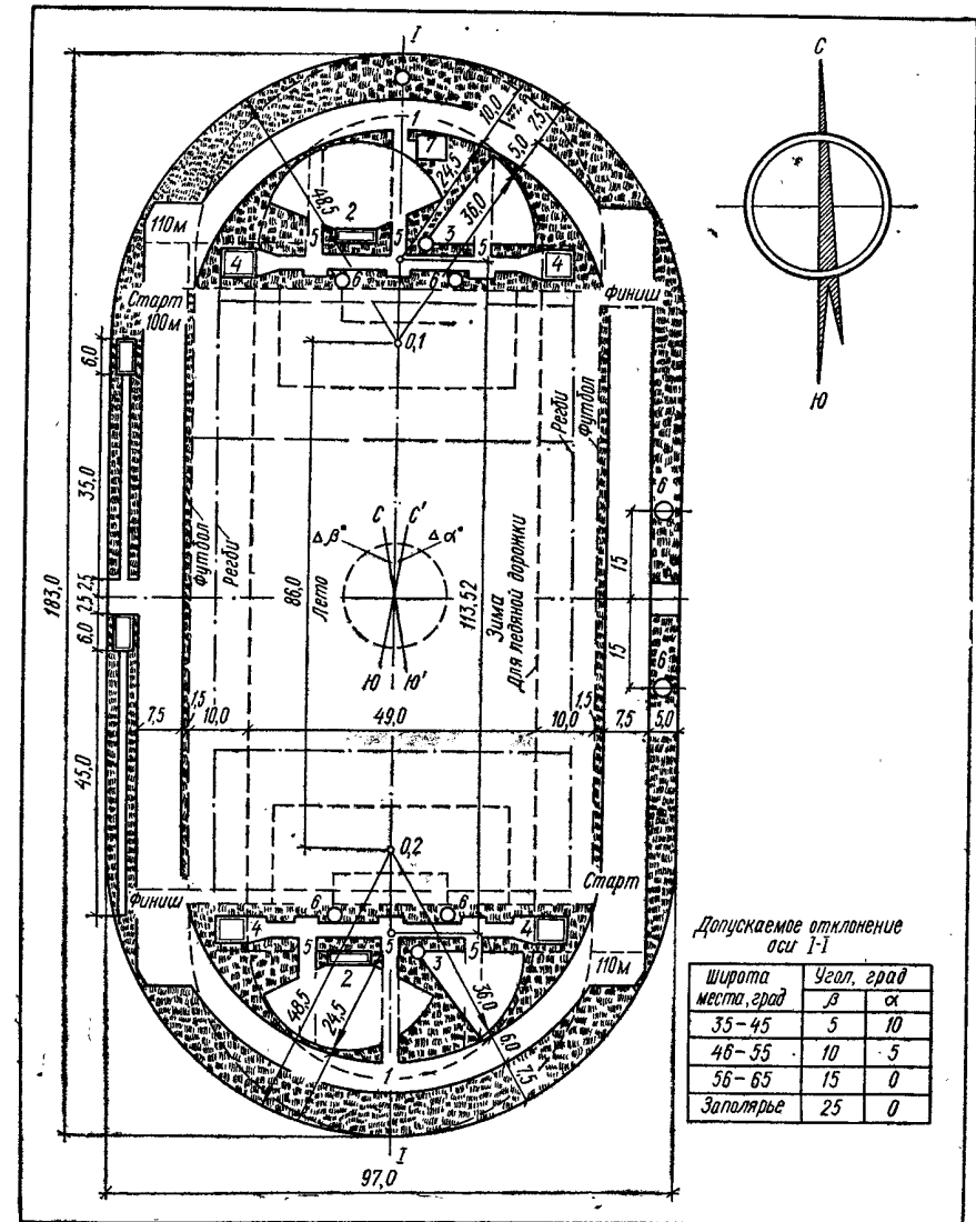
Рис. VIII.2. Пример планировки спортарены для малых стадионов: 1 — беговая дорожка 400 м; 2 — место для прыжков в высоту; 3 — толкание ядра; 4 — прыжки в длину, тройной и с шестом; 5 — метание копья; 6 — метание диска; 7 — яма с водой; \alpha, \beta — углы отклонения продольной оси от географического меридиана.
