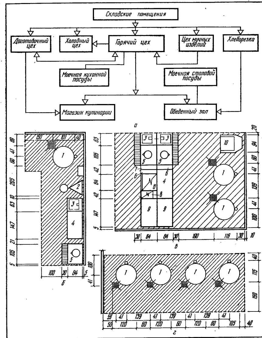
Рис. VII.58. Взаимосвязь производственных помещений и функциональные зоны приготовления первых блюд: а — функциональная взаимосвязь производственных помещений; б — зона приготовления первых блюд в столовой на 100 мест; в — зона приготовления первых блюд и гарниров в столовой на 150 мест; г — зона стационарных котлов для приготовления первых блюд и гарниров в столовой на 300 мест; 1 — котел пищеvarочный электрический; 2 — универсальный привод общего назначения; 3 — ванна моечная передвижная; 4 — стол для установки средств малой механизации; 5 — котел пищеvarочный секционный модулированный; 6 — секция-вставка к тепловому оборудованию с краном-смесителем; 7 — секция-вставка к тепловому оборудованию с гладким столом; 8 — плита электрическая секционная модулированная; 9 — стол производственный; 10 — машина для приготовления картофельного пюре.
