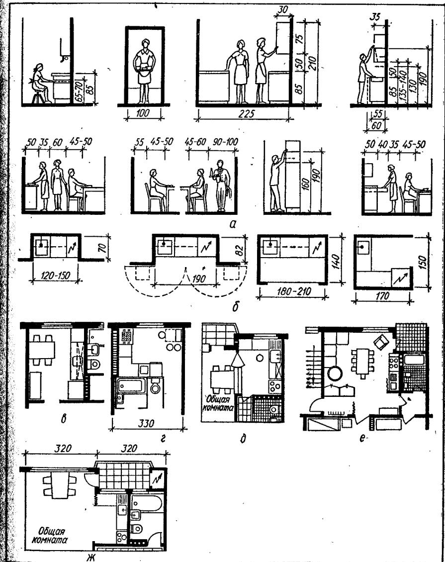
Рис. VI.15. Габариты и оборудование кухни
