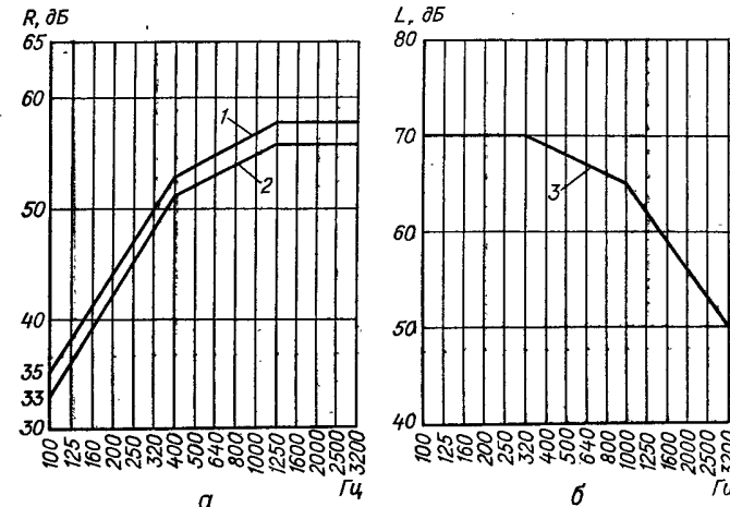
Рис. II.21. Нормативные кривые частотных характеристик звукоизолирующей способности ограждения:
