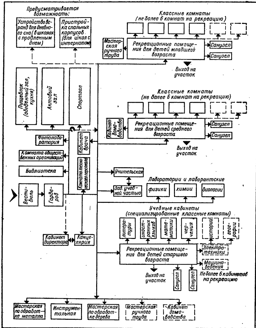
Рис. VII.9. Организационная структура и функциональная взаимосвязь помещений общеобразовательных школ и школ-интернатов (пунктиром показаны дополнительные связи между помещениями и возможные группировки помещений).
