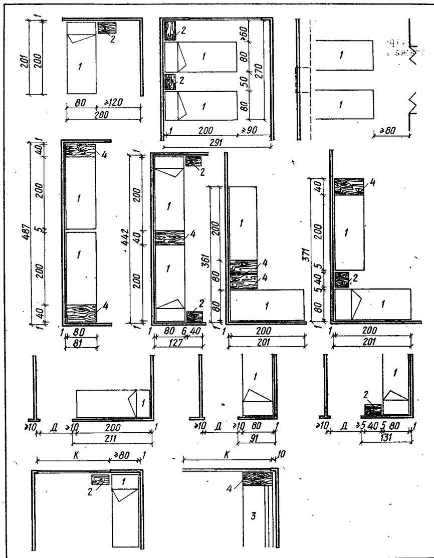
Рис. VI.34. Нормированные расстояния при группировке мебели для сна в гостиницах:
