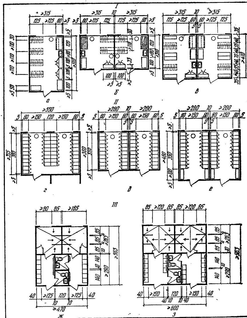
Рис. VII.111. Габаритные схемы обслуживающих помещений в пионерских лагерях: I — гардероб-вещевые отряды при хранении одежды на открытых вешалках; II — то же, в индивидуальных шкафчиках; III — душевые; a , б — на 40 человек; в , г , е — на 20 X 2 = 40 человек; ж — на 6 сеток в лагере вместимостью до 240 мест; з — на 10 сеток в лагере вместимостью более 240 мест.
