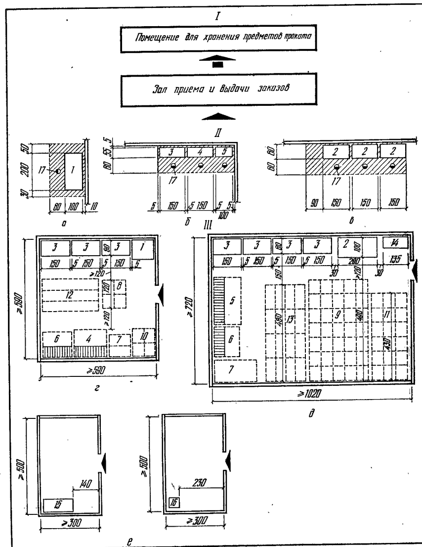
Рис. VII.69. Примеры и элементы планировки пунктов проката:
