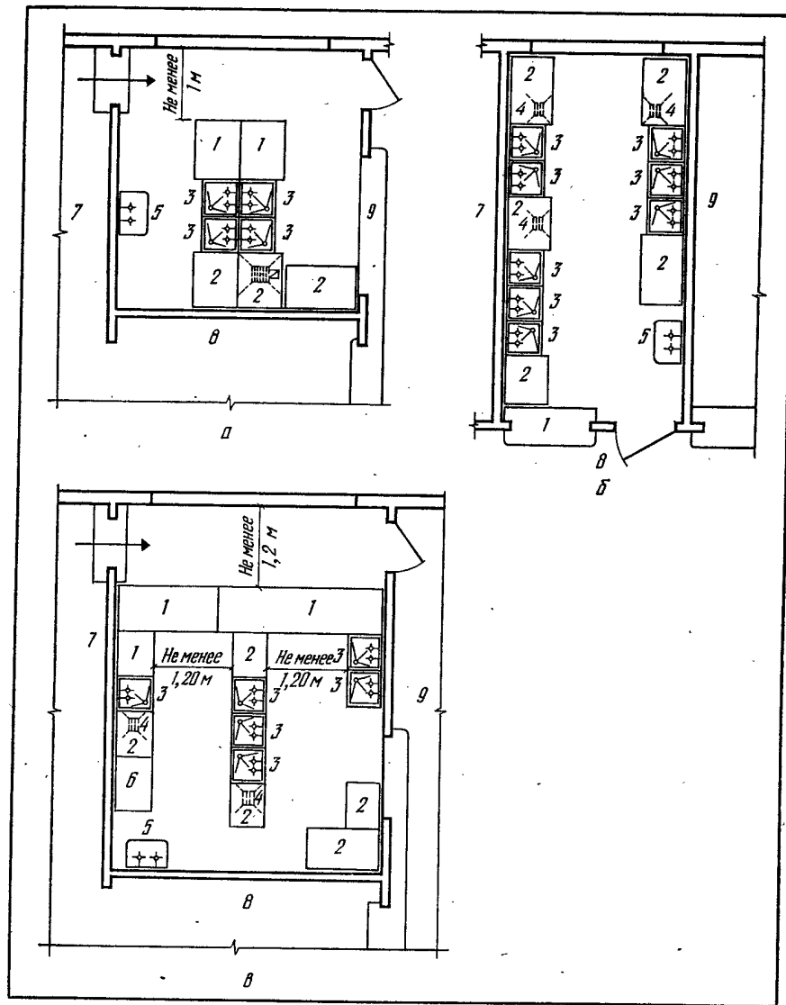
Рис. VII.57. Варианты планировки моечных столовой посуды: а — с двумя потоками; б, в — с тремя потоками; 1 — приемный стол; 2 — рабочий стол; 3 — ванна; 4 — трап; 5 — раковина; 6 — шкаф для посуды; 7 — обеденный зал; 8 — раздаточная; 9 — кухня.
