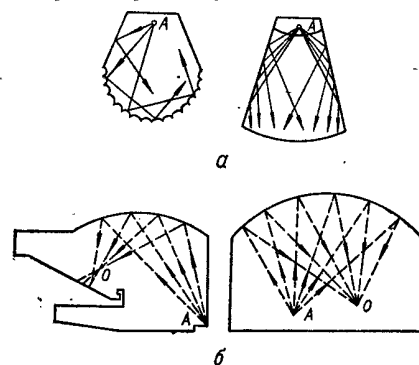
Рис. II.17. Схемы отражений звуковых лучей в залах: а — от стен; б — от потолков
