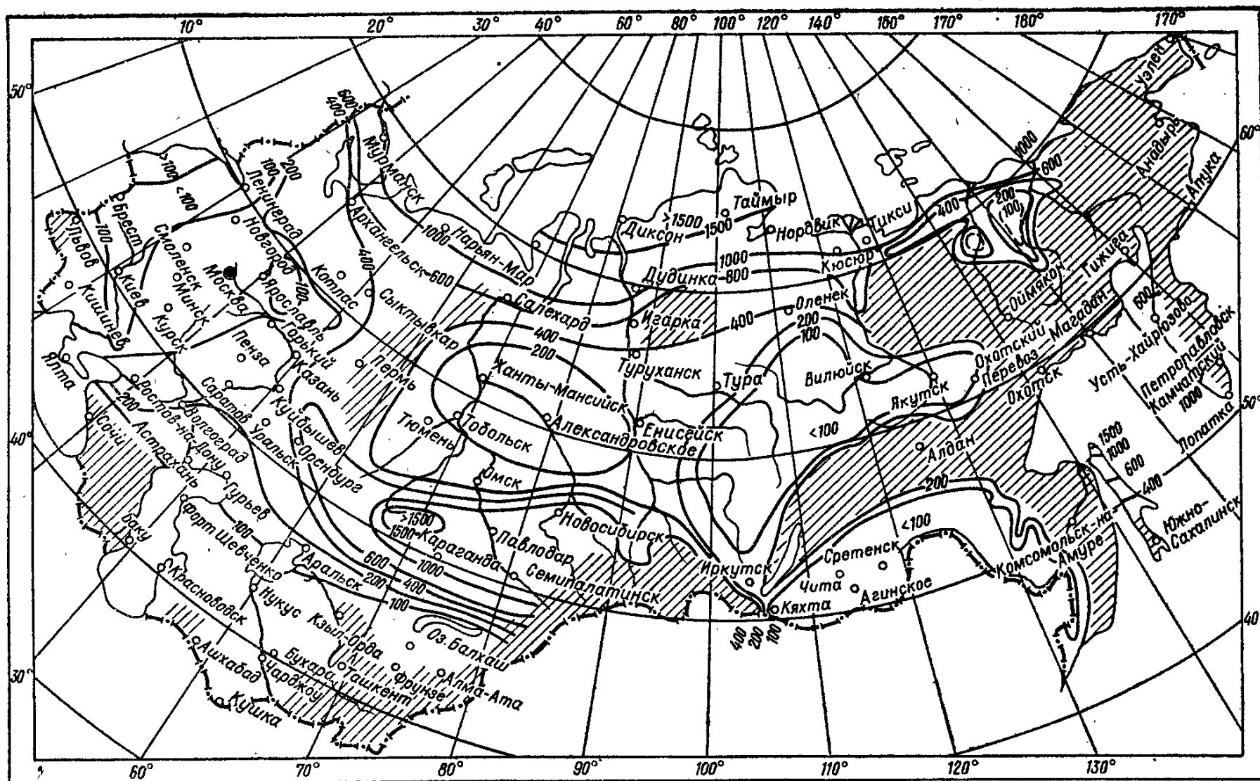
Рис. 1.6. Схематическая карта СССР по объемам максимального снегопереноса за зиму при общих и низовых метелях, \text{м}^3/\text{м} .
