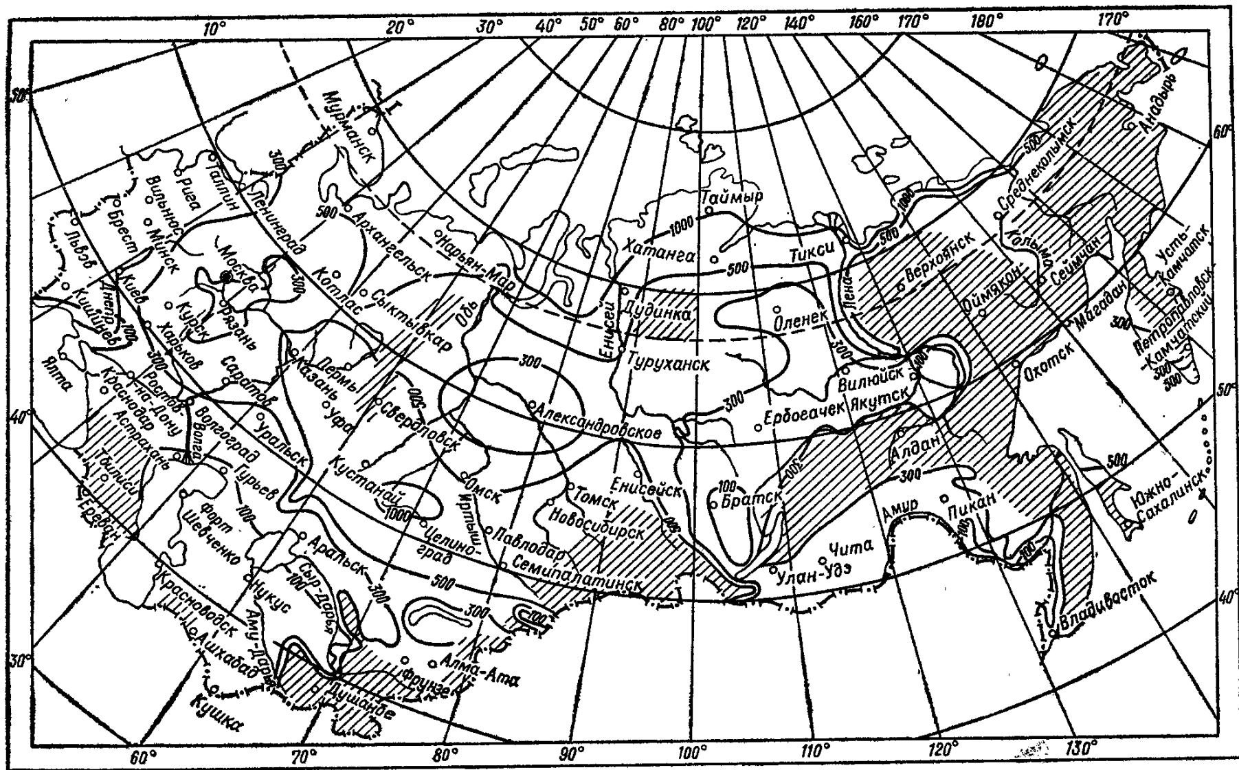
Рис. 1.5. Схематическая карта СССР максимальной за зиму продолжительности переноса снега при общих и низовых метелях, ч.
