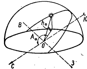
Рис. II.9. Схема параметров траектории движения солнца по небосводу:
