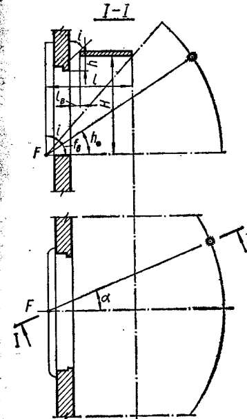
Рис. 11.15. Схема к расчету выноса горизонтального козырька: l — общий вынос козырька; l_b — размер воздушного зазора между козырьком и стеной.
