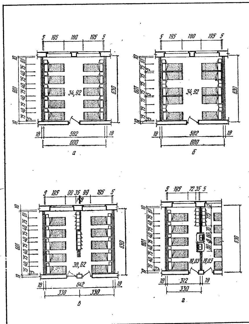
Рис. VII.109. Примеры и габаритные схемы планировки спальных помещений:
