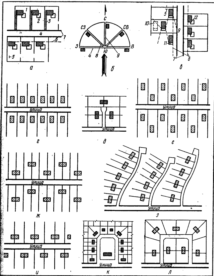
рис. VI.35. Размещение домов по условиям ориентации и схемы организации приквартирных участков: а — при широтном направлении улицы; б — оптимальное расположение домов при различном направлении улиц; в — при меридиональном направлении улицы; г, и — обычное рядовое расположение домов; д — тупиковое расположение домов; е, ж — двухрядное расположение домов; з — тупиковое расположение на рельефе; к — расположение с открытой площадкой; л — расположение по внутреннему петлеобразному проезду; 1 — двор; 2 — терраса; 3 — подъезд; 4 — улица широтного направления; 5 — отступ от границы; 6 — линия застройки; 7 — красная линия; 8 — диагональная улица; 9 — улица меридионального направления; 10 — дом с наилучшим расположением; 11 — терраса, расположенная на юг; 12 — то же, на юго-восток.
