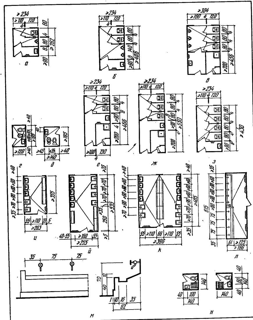
Рис. VII.113. Габаритные схемы санитарных узлов в пионерских лагерях:
