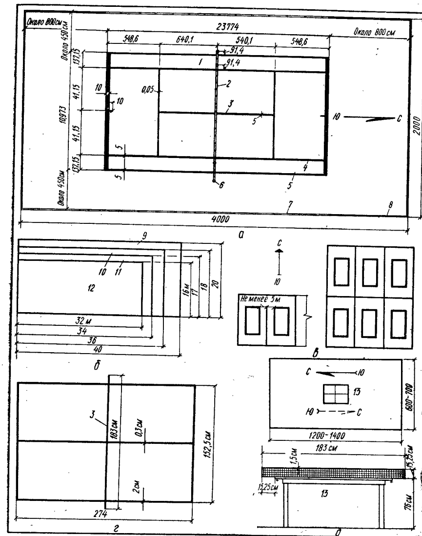
Рис. VIII.4. Теннисная площадка: а — план; б — размеры площадки для настольного тенниса; в — блокировка; г — разметка; д — настольный теннис; 1 — подпорка; 2 — сетка; 3 — средняя линия; 4, 5 — боковая линия для игры соответственно одиночной и парной; 6 — стойка (столб); 7, 8 — ограждение не менее соответственно 1 и 3 м; 9 — для соревнований; 10 — для городских спортцентров; 11 — для жилых районов; 12 — для микрорайонов; 13 — теннисный стол с сеткой.
