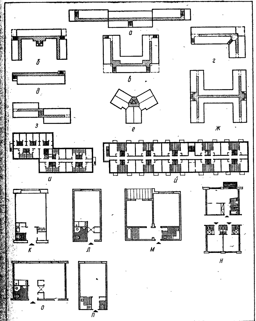
Рис. VI.5. Компонка планов домов гостиничного типа (а—г) и планы секций (к—п): а, б — по коридорно-галерейной схеме; в, д — по галерейной схеме; ж, з, е — з — по коридорной схеме; и, й — типовые этажи; к, л, о, п — секции 1-комнатных квартир; м — секция 2-комнатной квартиры; н — компоновка секций 2-комнатных квартир.
