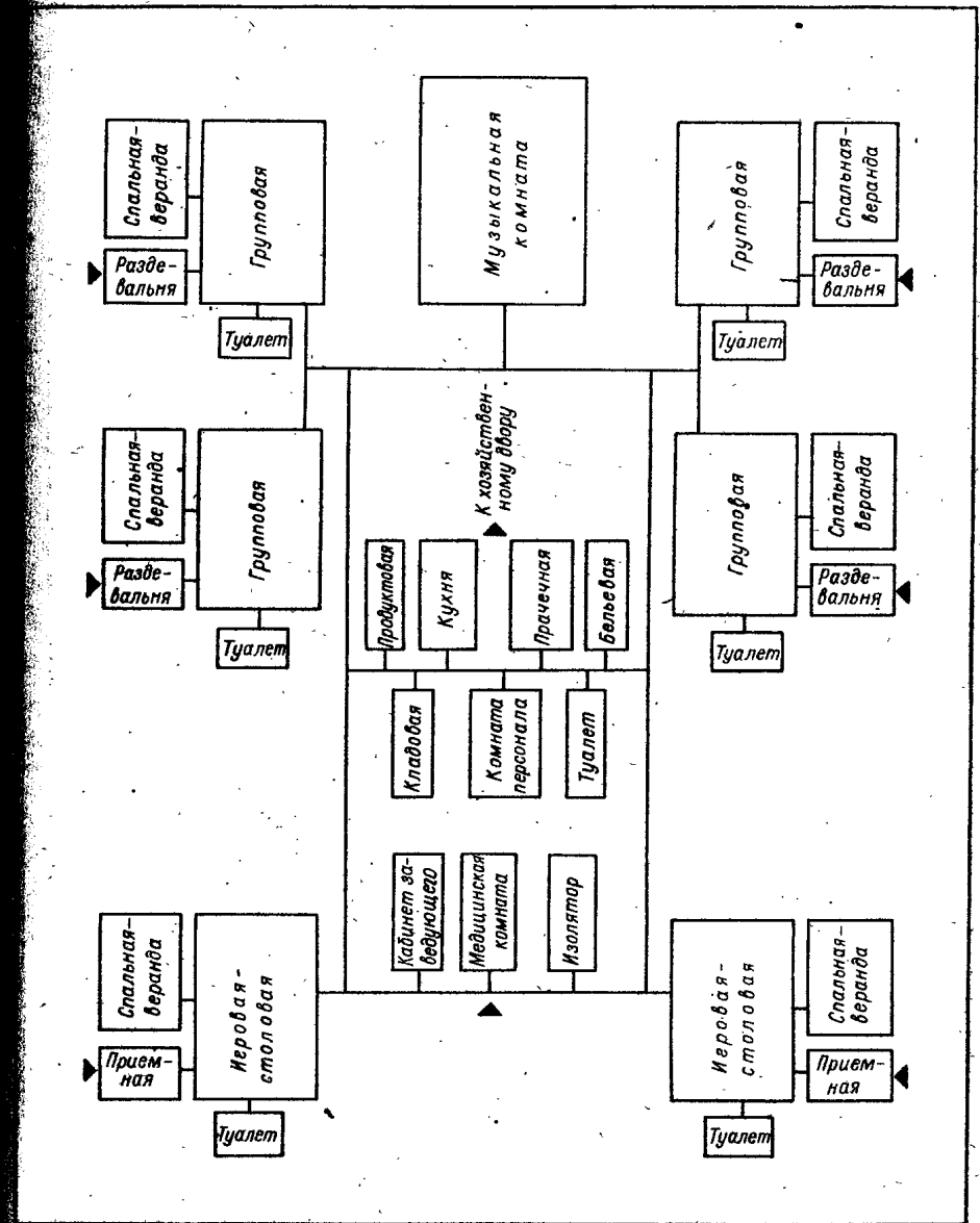
Рис. VII.3. Функциональная взаимосвязь помещений круглосуточных яслей-сада на 140 мест.
