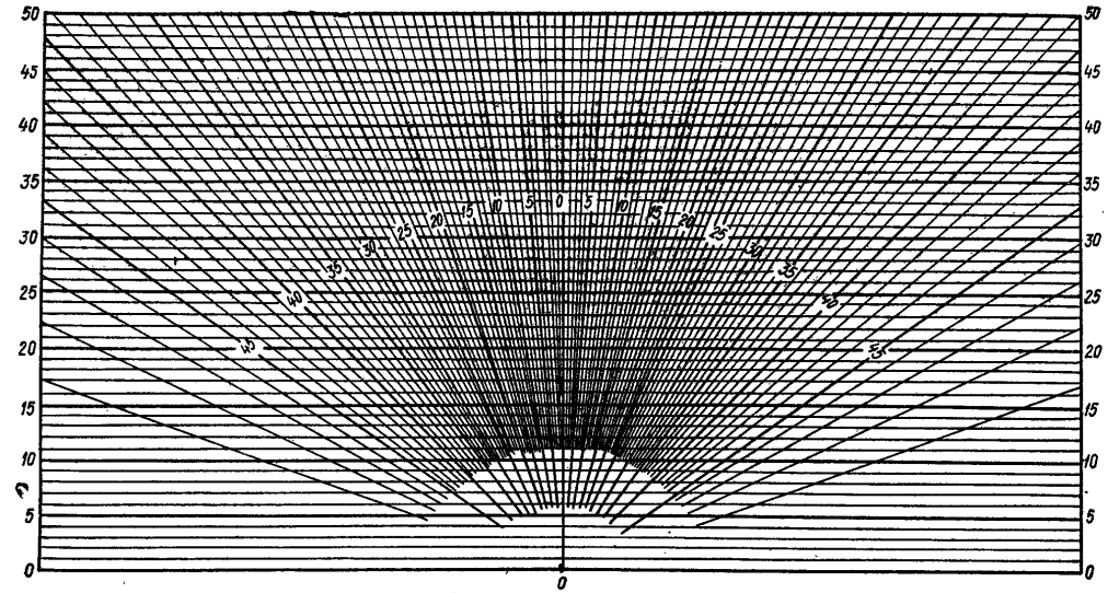
Рис. 11.6. График II А. М. Данилюка для расчета геометрических коэффициентов освещенности при боковом и верхнем освещении \epsilon_6 и \epsilon_в .
