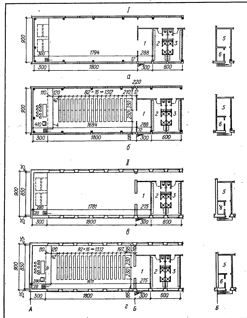
Рис. VII.18. Планировка гимнастических и актов залов в одних и тех же габаритах в зданиях школ конструкций:
