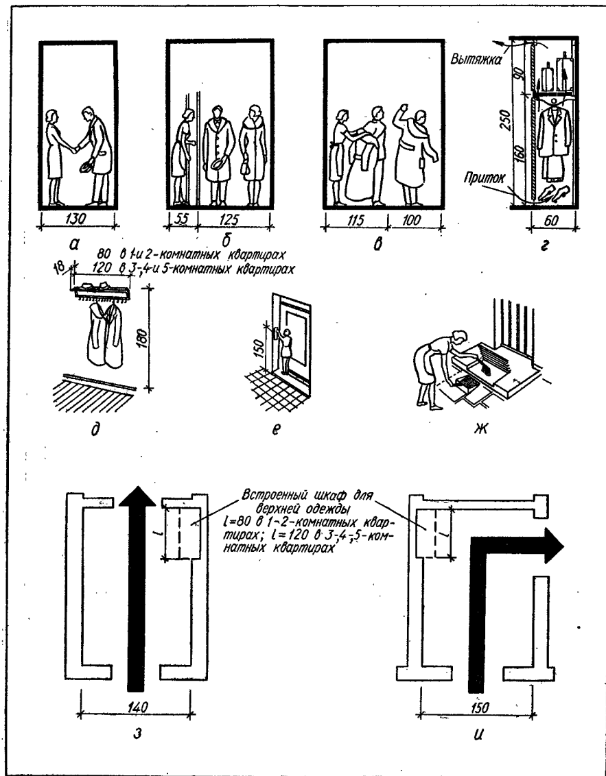
Рис. VI.14. Габариты (минимальные) и оборудование передней;
