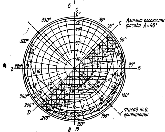
Рис. II.14. К примеру определения продолжительности инсоляции при f_T = 180^\circ : а — схема вертикальных углов затенения ( f_B = 28^\circ ) противостоящим зданием; f_B = 52^\circ — нависающим балконом; f_B = 72^\circ — верхом окна; б — вспомогательный график с нанесенными зонами затенения; в — от здания, при f_B = 28^\circ ; Б — от балкона при f_B = 52^\circ ; Г — от верха окна при f_B = 72^\circ и f_T = 160^\circ ; в — совмещение подготовленного вспомогательного графика с солнечной картой Дунаева для 50° с. ш. Ориентация фасада Ю = З. А \odot = 135^\circ .
