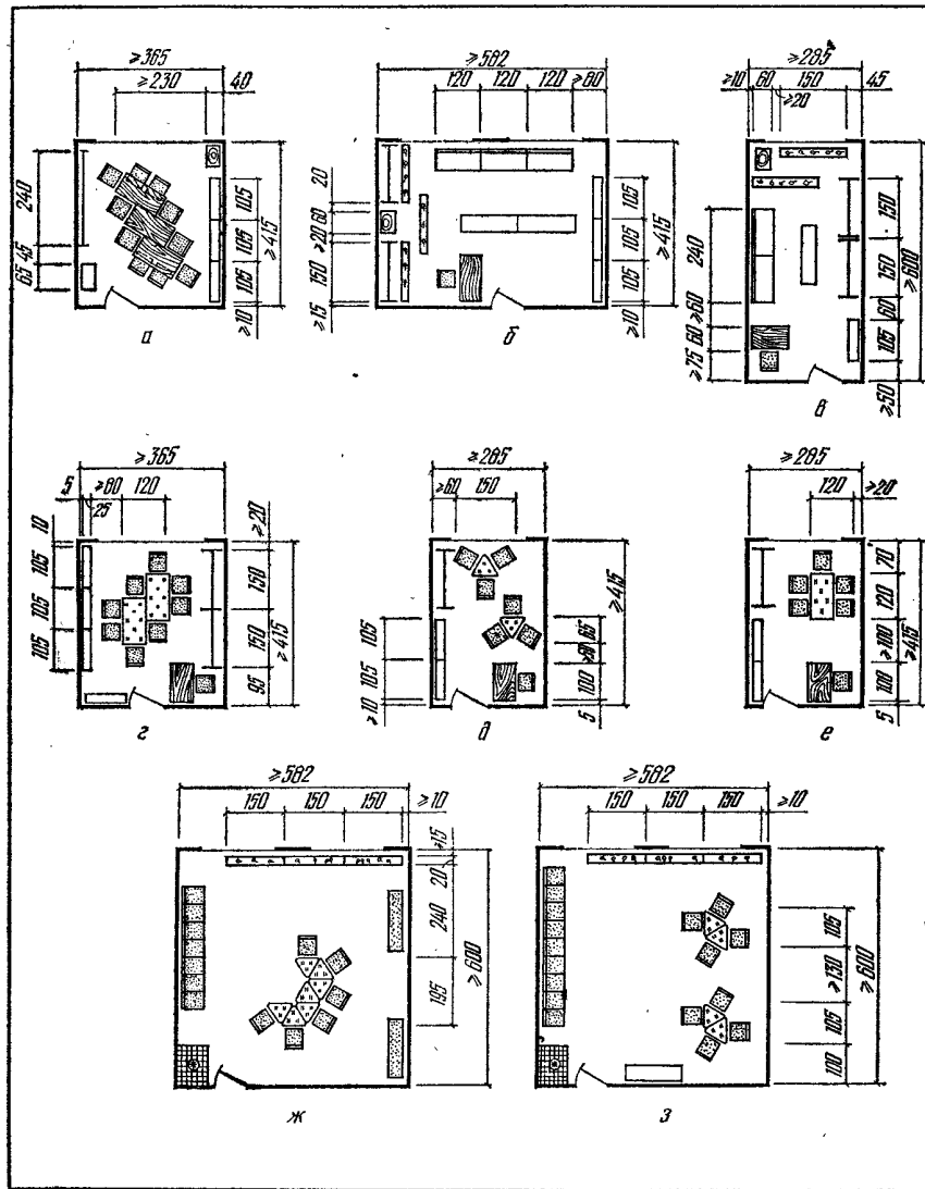
Рис. VII.112. Габаритные схемы помещений культурно-массового обслуживания пионерских лагерей:
