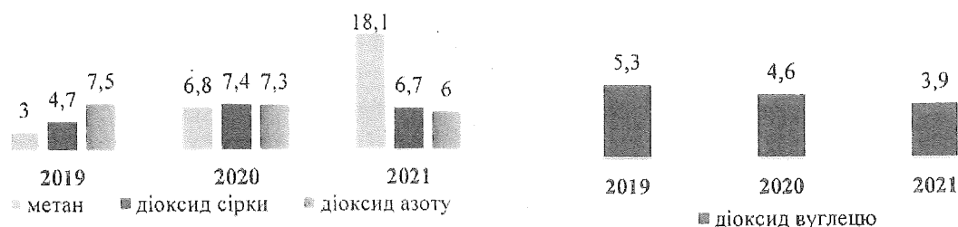
Рисунки 2. Динаміка викидів метану, діоксиду сірки, діоксиду азоту, тис. т
