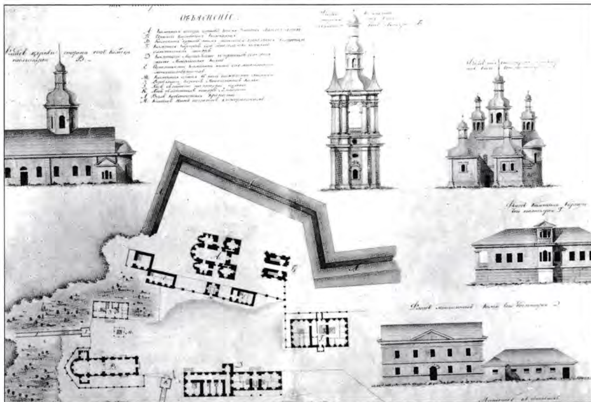
Києво-Печерська лавра. Споруди ансамблю Дальніх печер. Обмірні кресленики архітектора А. Меленського 1820-х рр.
